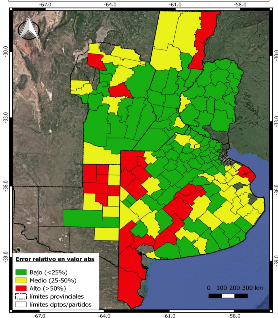
Figura 1. Mapa de acuerdo para el índice de variación interanual de maíz entre el producto AMZ y las series estadísticas de Estimaciones Agrícolas – MAGyP.
