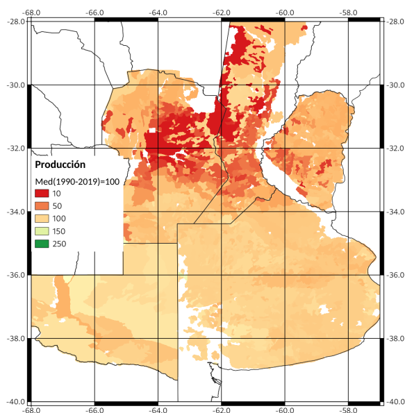
Figura 1. Mapa de anomalías para la mediana de los escenarios de rinde de trigo pronosticadas el día 25 de julio de 2020 para el final de la campaña tomando como base un producción normal. El año normal se corresponde con el valor de la mediana de los rindes calculados entre 1990 y 2019. EL mapa fue generado a través del procesamiento por ZH sobre la Región Pampeana.
